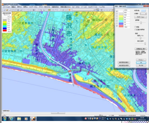
← 図5 標高データの色分けの表現を工夫する
